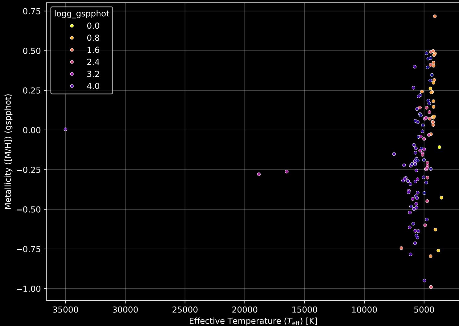
APOGEE DR17 Field: [279-32-O_TESS] Stellar Population Parameters (n= 122)
